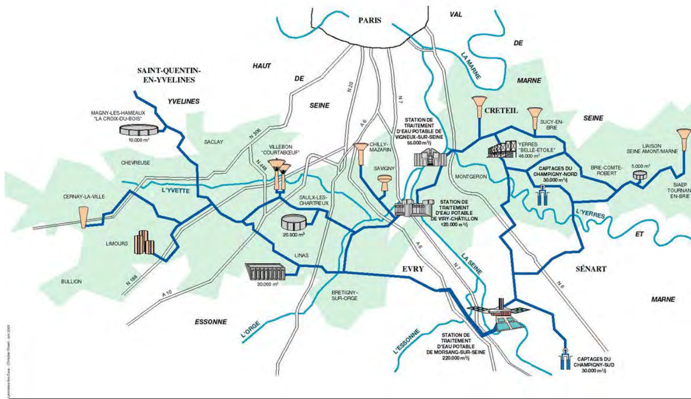
RÉSEAU INTERCONNECTÉ DE LYONNAISE DES EAUX AU SUD DE LA RÉGION PARISIENNE
